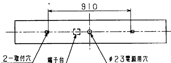
取付寸法図
