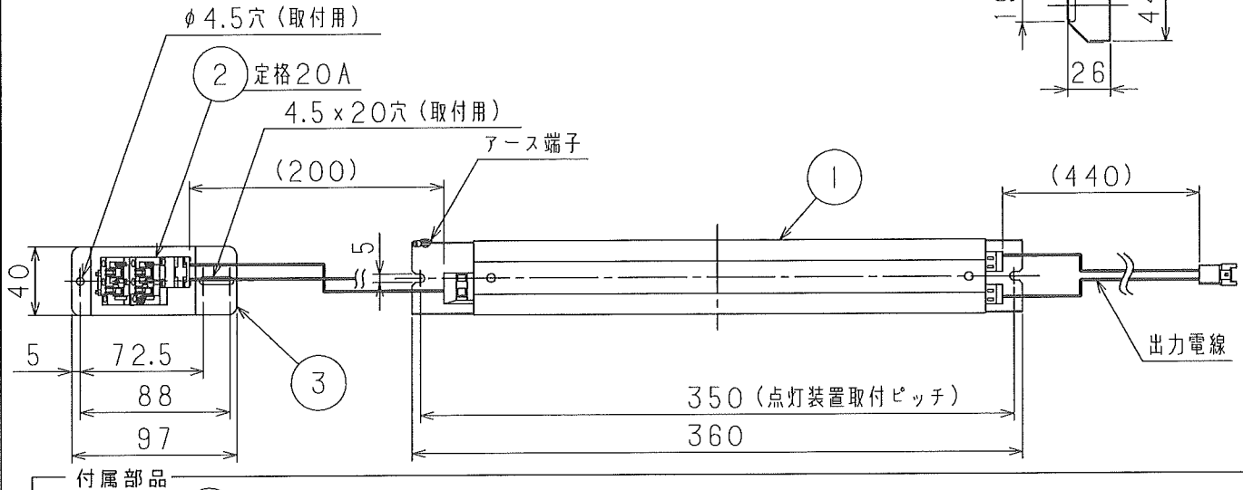
付属部品
