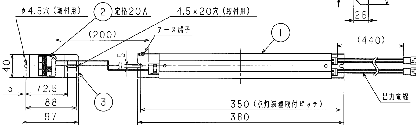
付属部品
