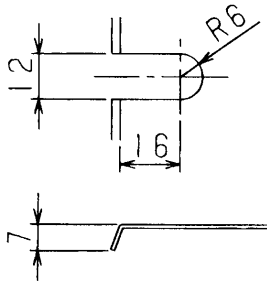
取付穴詳細
