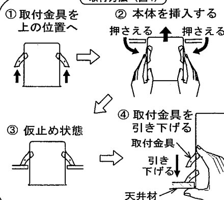
取付方法(図4)
