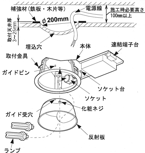
速結端子台線の接続と解除(図1)
