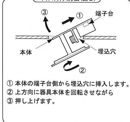
本体の挿入方法(図2)
