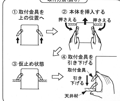
取付方法(図3)
