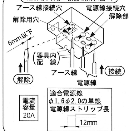
速結端子台線の接続と解除(図1)
