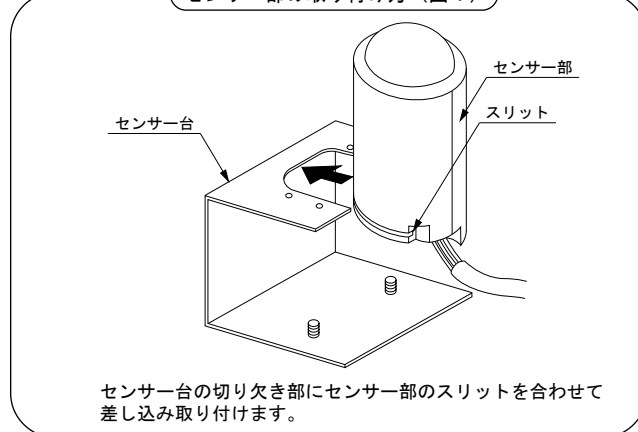
センサー部の取り付け方（図1）
