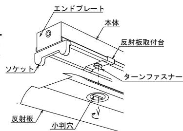
反射板の取付方法 (図7) 図例は2灯用です
