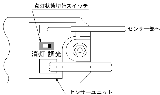
点灯状態設定スイッチ部 (図6)
