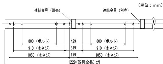
連結のしかた (図3)
