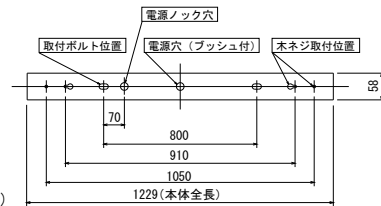
器具質量と背面取付穴 (図2)
