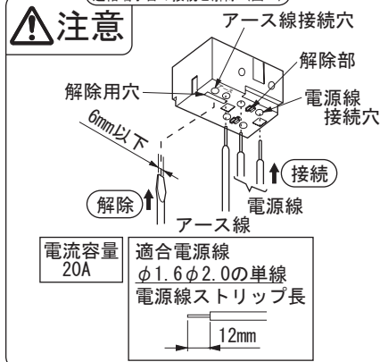
連結端子台の接続と解除 (図3)
