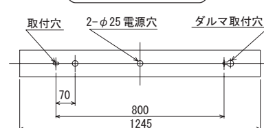
背面取付穴 (図1)
