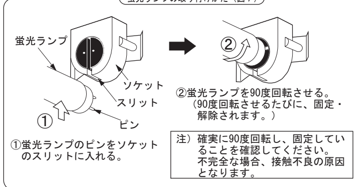
蛍光ランプの取り付けかた (図7)
