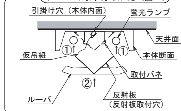
ルーバの取り付けかた (図6)
