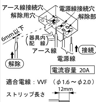
速結端子台の接続と解除(図3)
