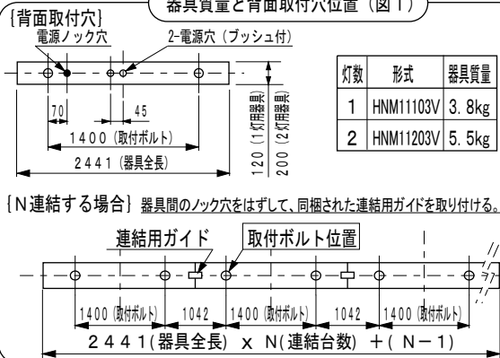
器具質量と背面取付穴位置（図1）
