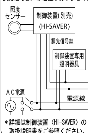
結線図
