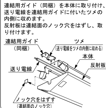
連結のしかた（図2）
