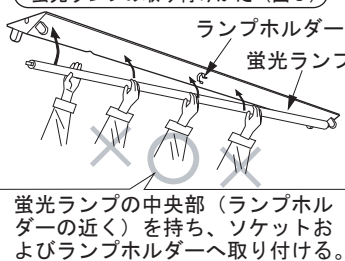
蛍光ランプの取り付けかた（図3）
