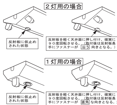
反射板取付方法（図４）
