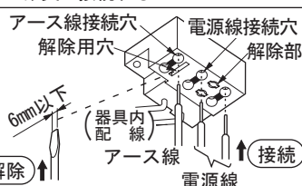
連結端子台の接続と解除（図2）
