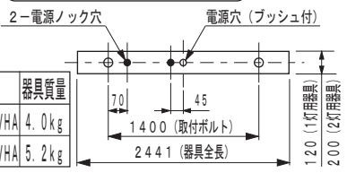
器具質量と背面取付穴（図1）
