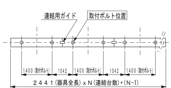
単体N連結する場合の取付ピッチ（図５）
