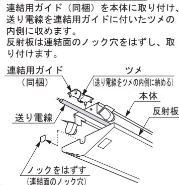
連結のしかた（図６）
