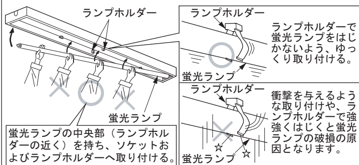
蛍光灯の取り付けかた（図４）
