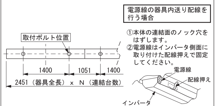
単体N連結する場合（図５）
