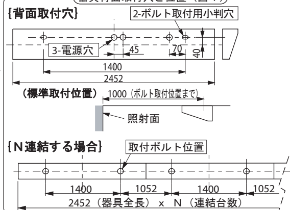
器具背面取付穴と位置(図1)
