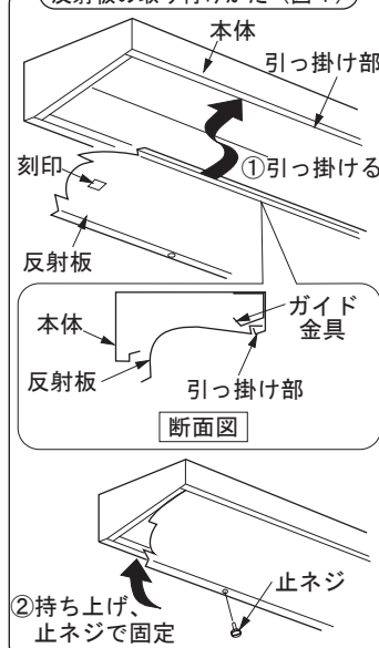
反射板の取り付けかた(図4)
