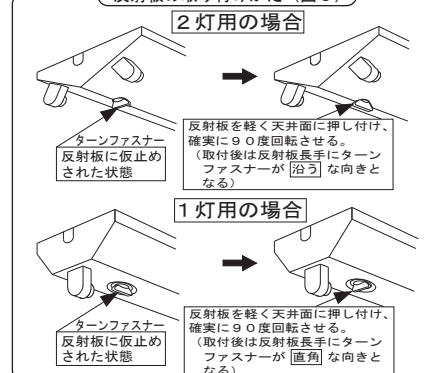
反射板の取り付けかた(図3)
