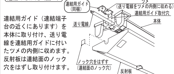
連結のしかた (図5)
