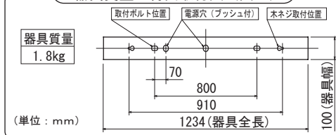
器具質量と背面取付穴(図1)
