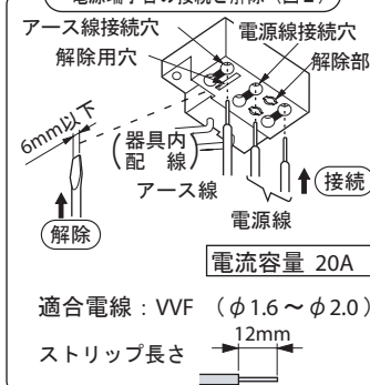
電源端子台の接続と解除(図2)
