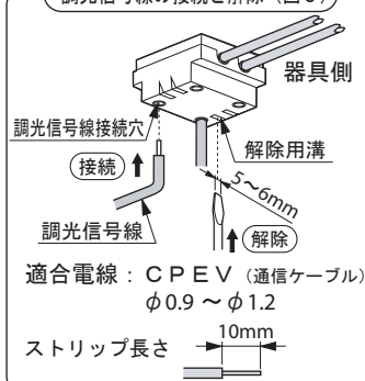
調光信号線の接続と解除(図3)
