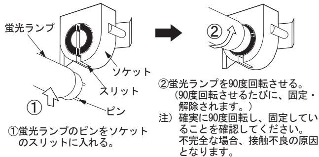
蛍光灯の取り付けかた（図4）
