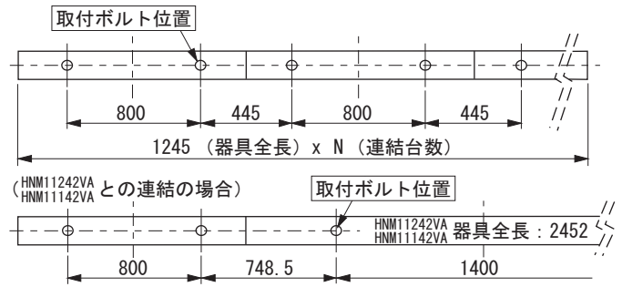
単体N連結する場合の取付ピッチ（図5）
