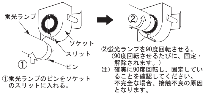
蛍光ランプの取り付けかた（図4）
