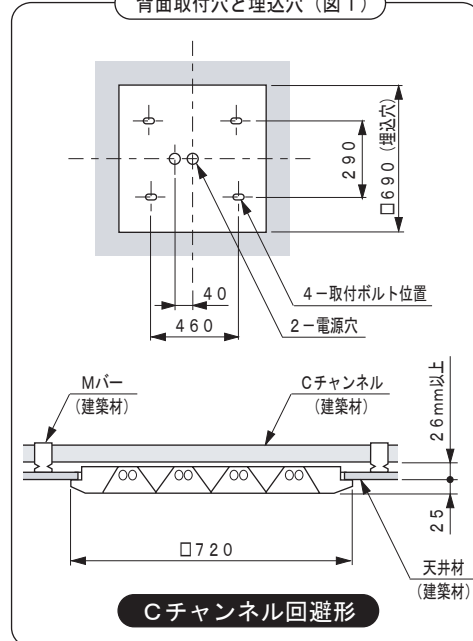
背面取付穴と埋込穴（図1）
