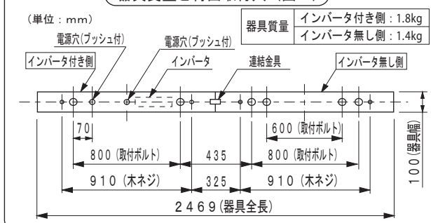
器具質量と背面取付穴(図1)
