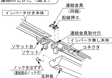
コネクタの接続と連結のしかた(図2)
