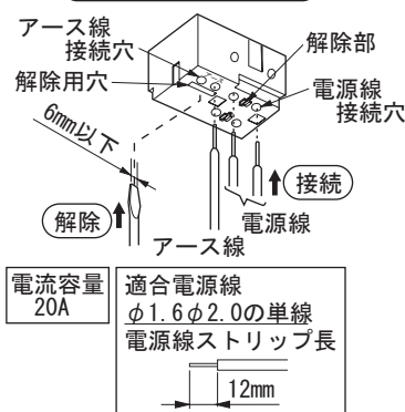
速結端子台の接続と解除 (図3)
