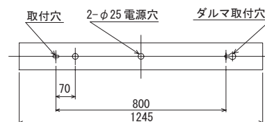
背面取付穴 (図1)
