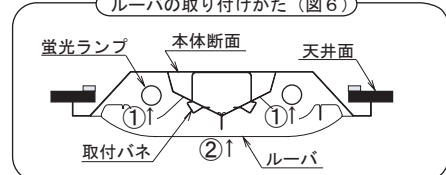
ルーバの取り付けかた (図6)
