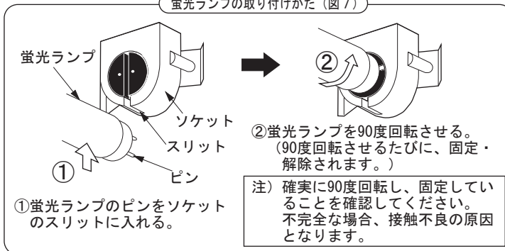
蛍光ランプの取り付けかた (図7)
