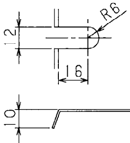
取付穴詳細
