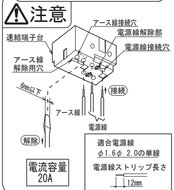
連結端子台の接続と解除(図3)
