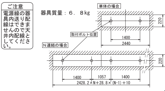
連結のしかた(図2)
