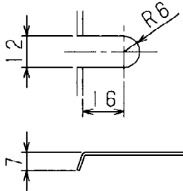
取付穴詳細
