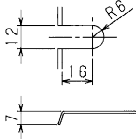
取付穴詳細
