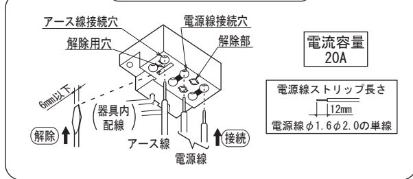
連結端子台の接続と解除 (図3)
