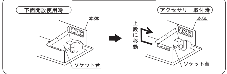
ソケット台の移動のしかた (図4)
