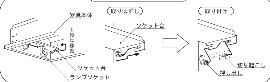
ソケット台の移動方法 (図3)
