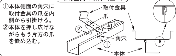
取付金具の取付 (図1)
