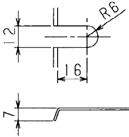
取付穴詳細
