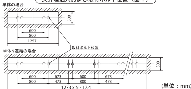
天井埋込穴および取付ボルト位置(図1)
