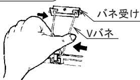
Vバネの取り付け(図3)
