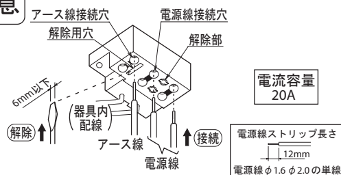
速結端子台の接続と解除(図2)
