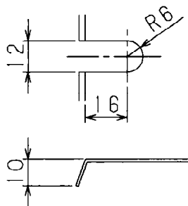
取付穴詳細
