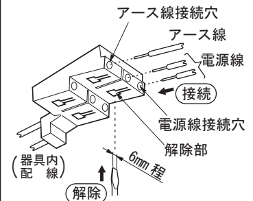
速結端子台の接続と解除(図3)
