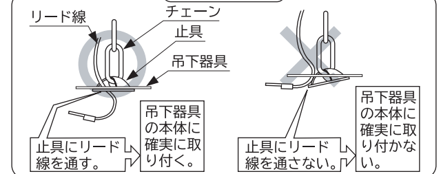
止具の確認(図3)
