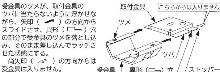
受金具の取り付け方(図2)
