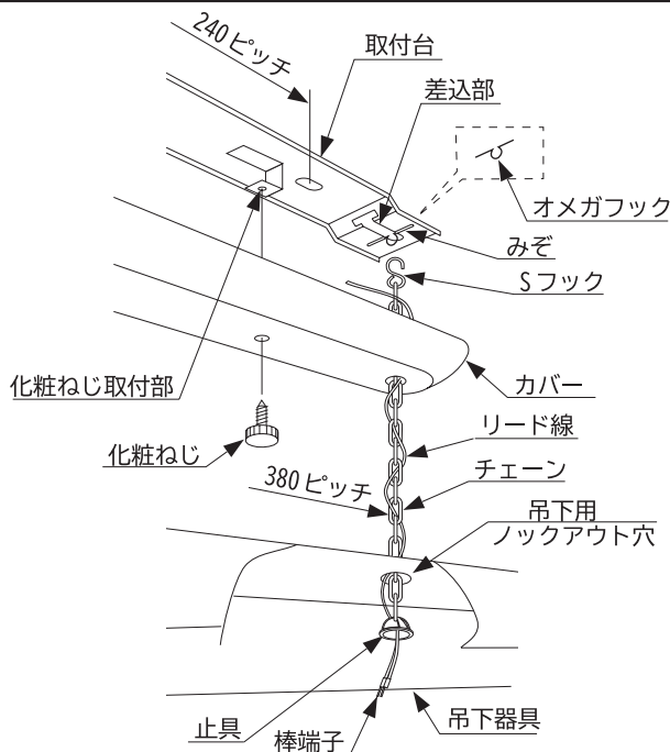
止具の確認(図2)
