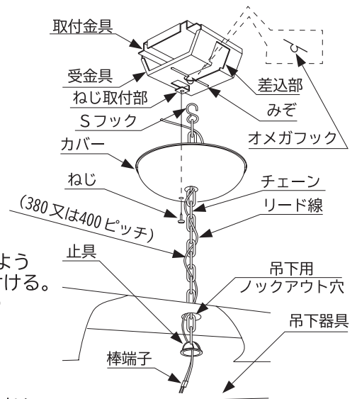
止具の確認(図3)
