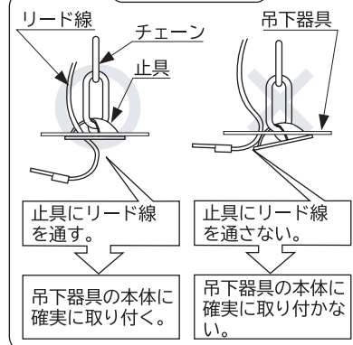
止具の確認(図2)
