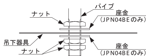
ナットの取り付けかた (図3)
