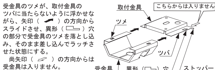
受金具の取り付けかた (図2)
