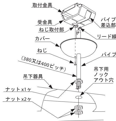
ナットの取り付けかた (図3)
