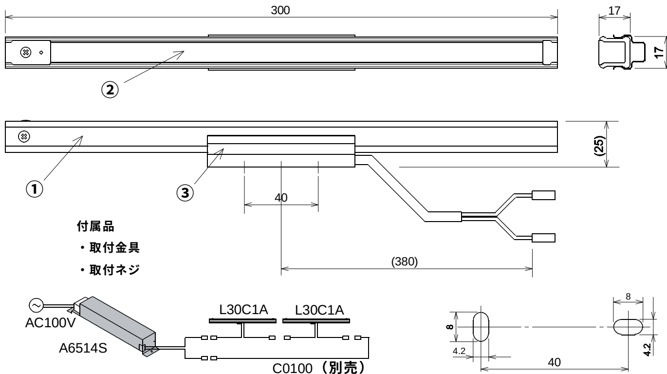
結線図（L30C1A×2台とA6514S×1台とC0100×1本の接続例）
