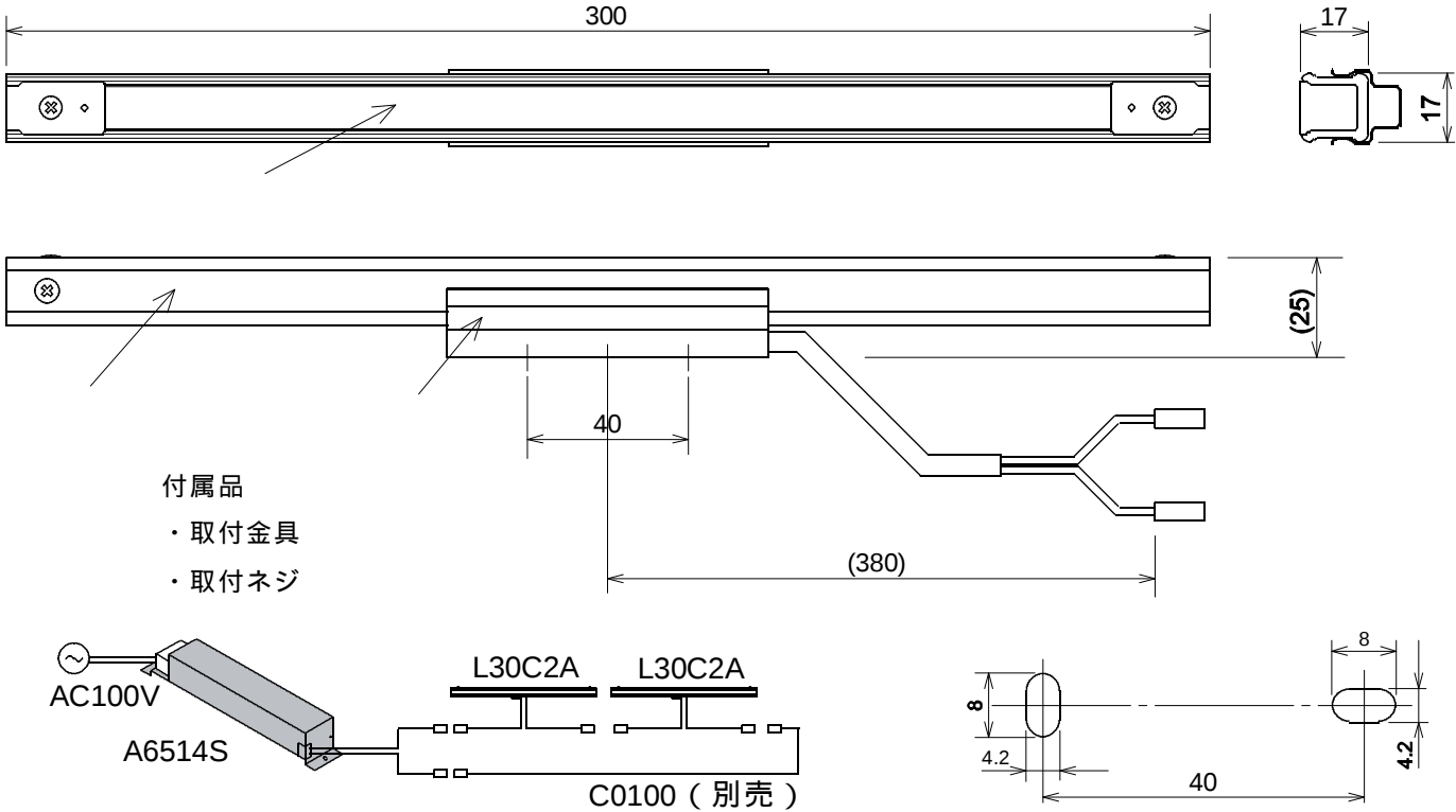
結線図（L30C2A×2台とA6514S×1台とC0100×1本の接続例）
