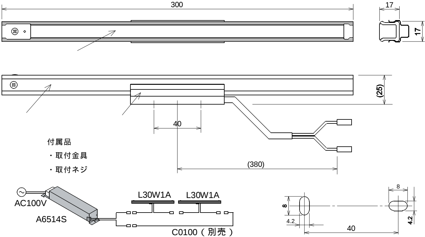
結線図（L30W1A×2台とA6514S×1台とC0100×1本の接続例）
