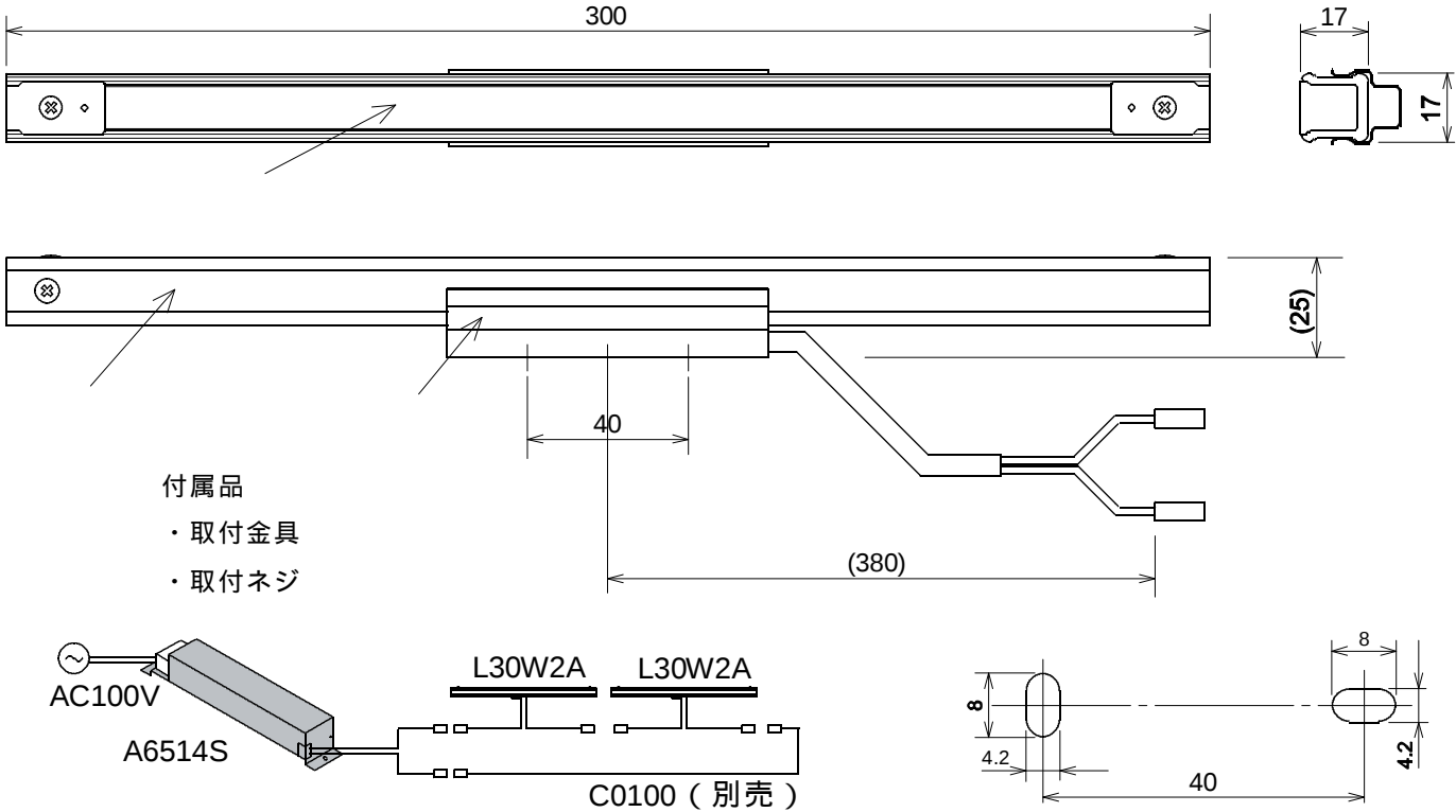
結線図（L30W2A×2台とA6514S×1台とC0100×1本の接続例）
