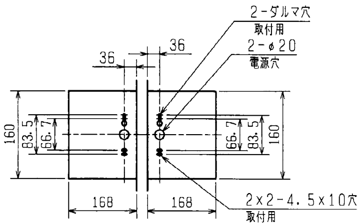
取付寸法図
