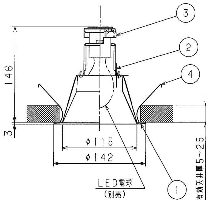
天井埋込穴寸法φ125
