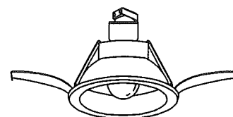
天井埋込穴寸法φ125
