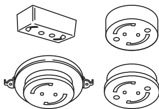
角形・丸形引掛シーリングボディ
