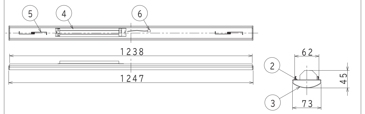
光源ユニット単体寸法図
