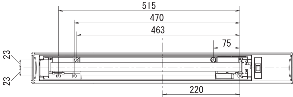
器具正面から見た取り付け穴位置
