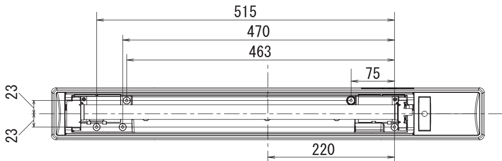
器具正面から見た取り付け穴位置
