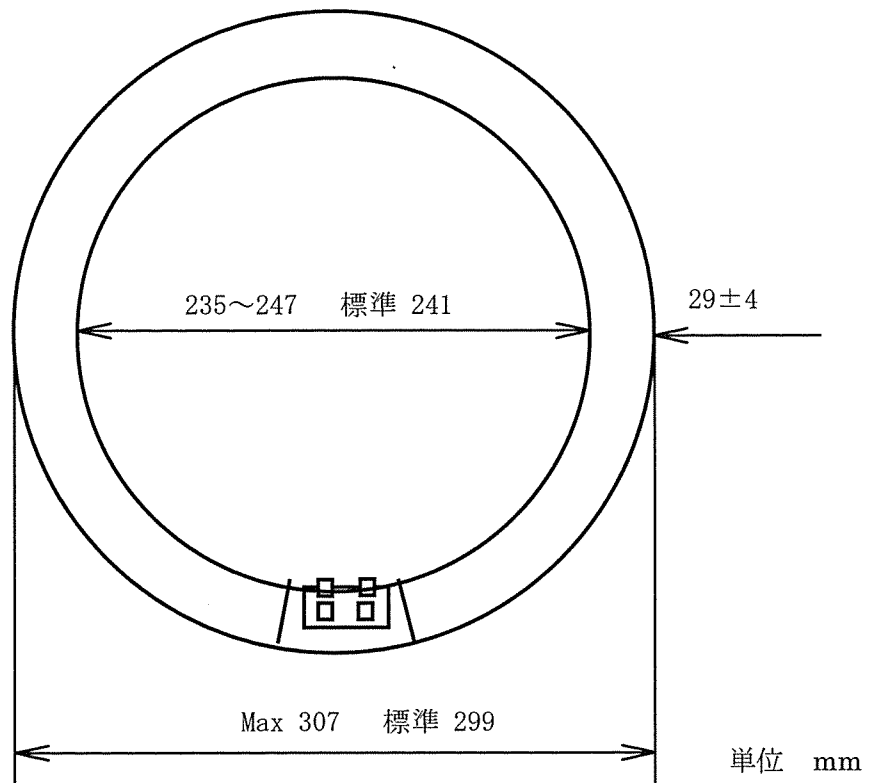
白色蛍光ランプ（環形）〈リングライト〉
