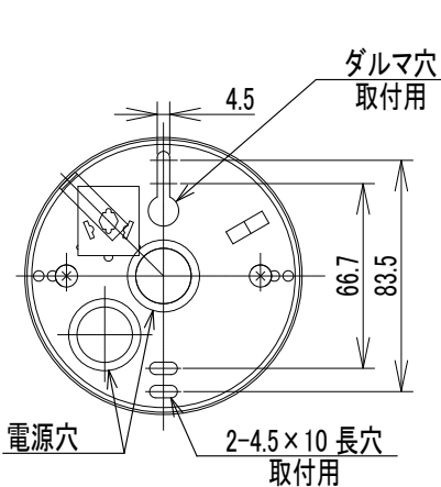
取付寸法図
