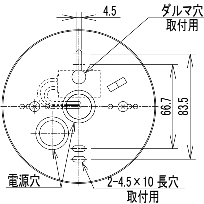
取付寸法図
