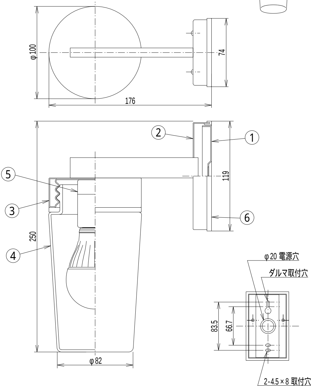
取付寸法図
