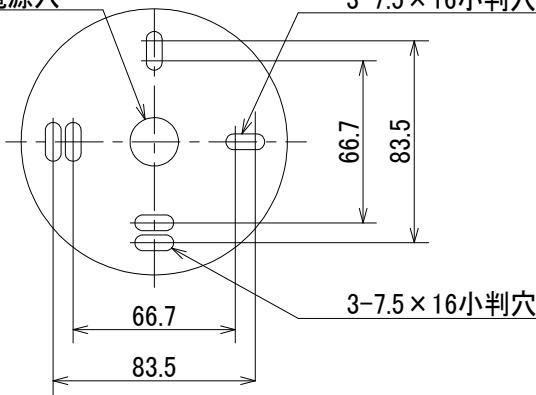
取付寸法図
